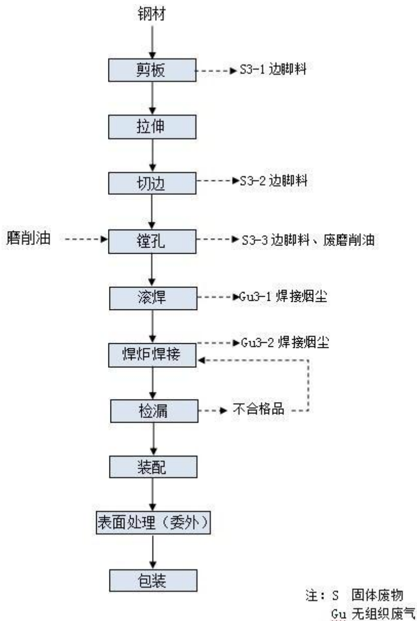
图 2-4 油箱工艺流程图
