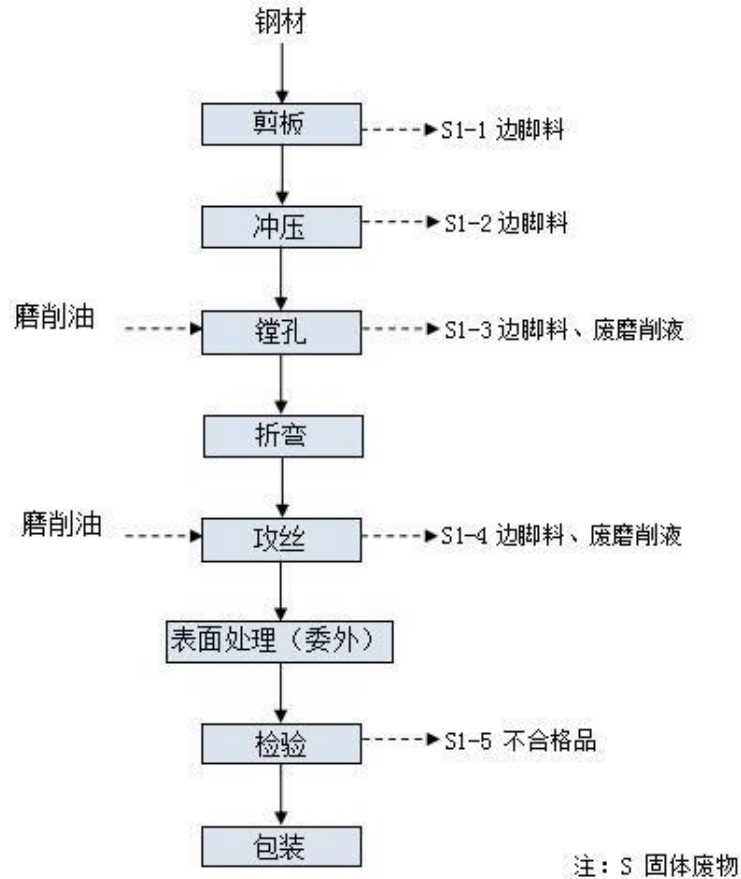
图 2-2 钣金件工艺流程图
