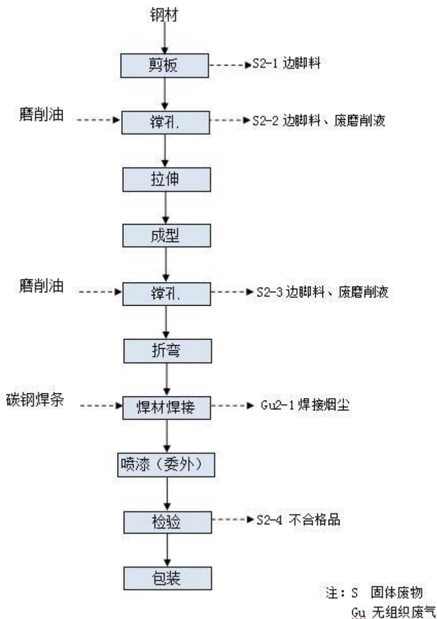
图 2-3 消声器工艺流程图
