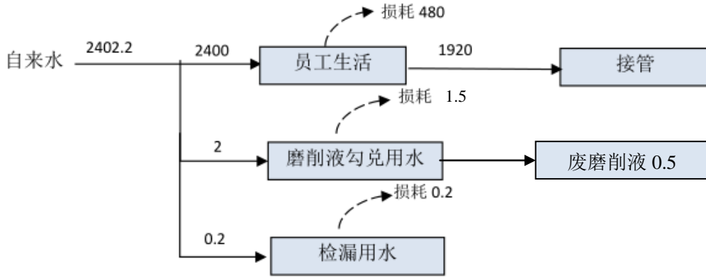
图 2-1 验收项目水平衡图 (t/a)
