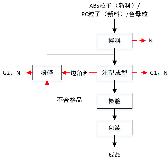
图 2-2 医疗器械零部件生产工艺流程图 (注: G n : 废气污染物; N: 噪声)
