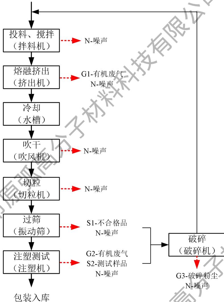
图 2-2 改性塑料粒子加工工艺流程图
