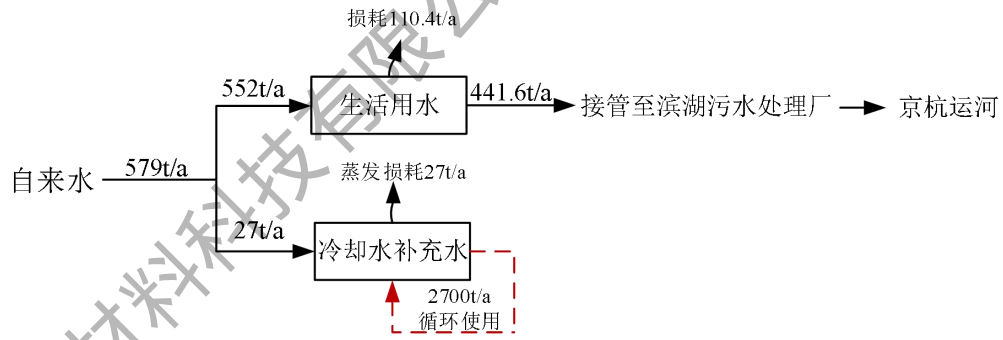
图 2-1 水平衡图
