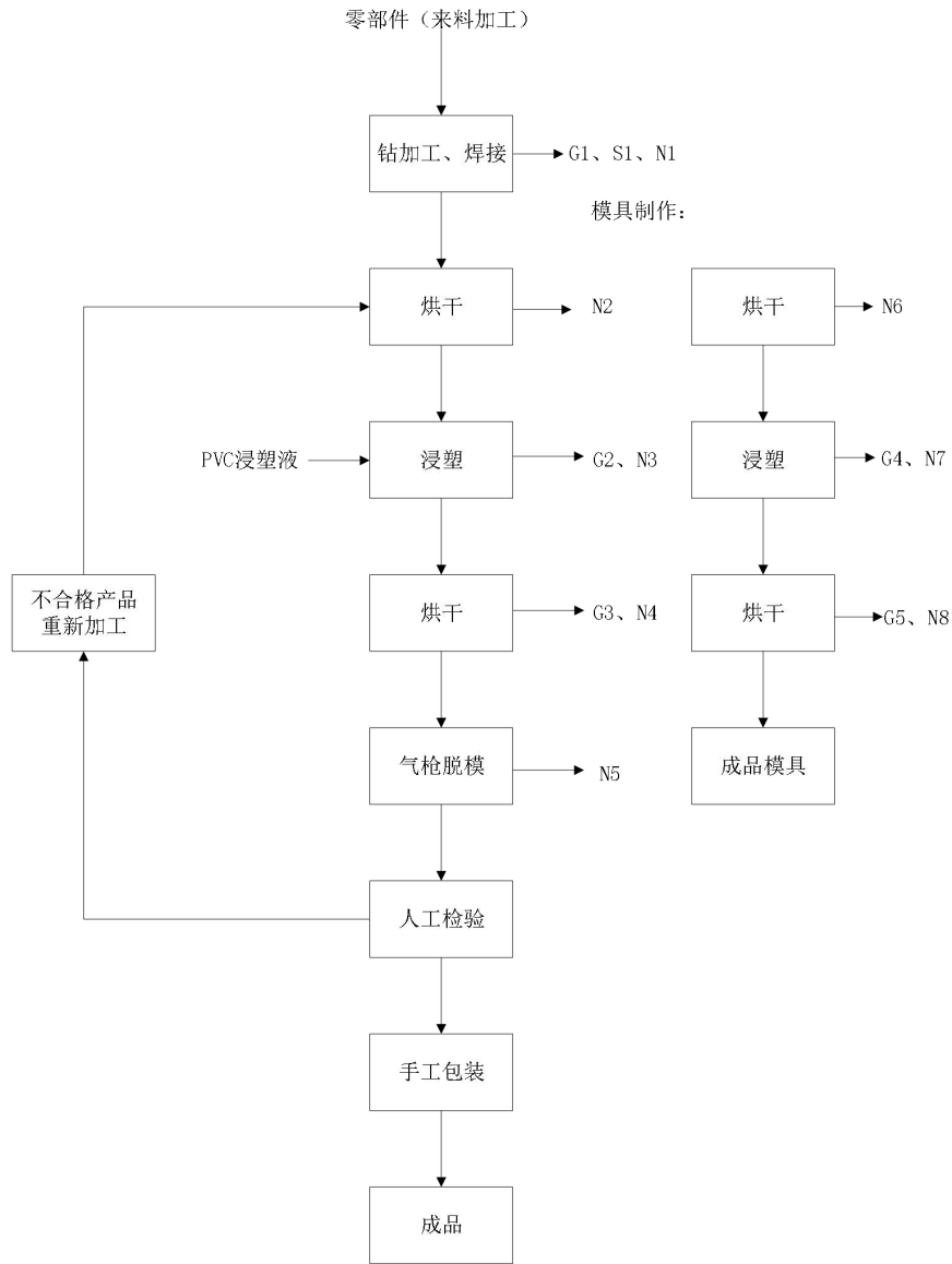
图 2-2 塑料柄套、塑料防护帽以及金属件包胶生产工艺流程图
